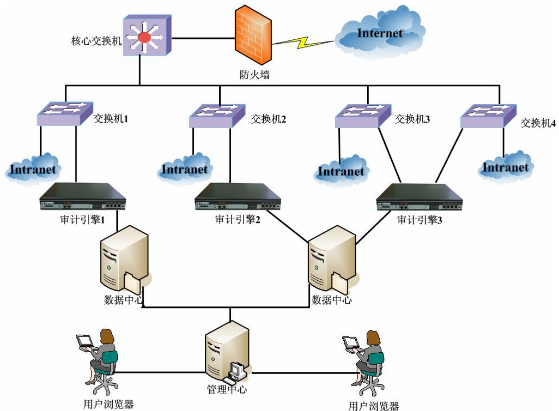
图 5-1 分布式部署方案示意图
